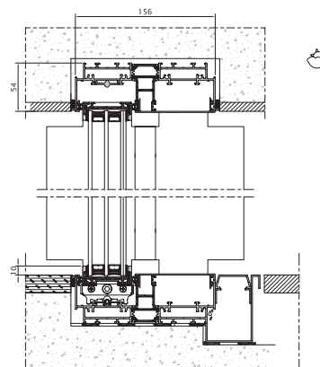
SEZIONE VERTICALE 2 ante - 1 anta mobile
