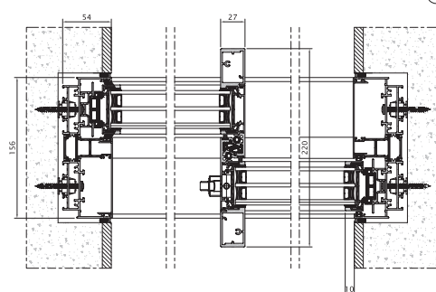
SEZIONE ORIZZONTALE 2 ante - 1 anta mobile
